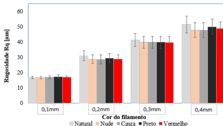
GRÁFICO 2. Resultados obtidos na rugosidade R_q para as diferentes alturas de camada.
