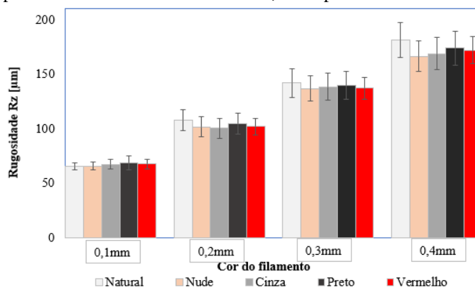
GRÁFICO 3. Resultados obtidos na rugosidade R_z para as diferentes alturas de camada.
