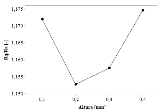
GRÁFICO 4. Relação Rq/Ra para as diferentes alturas de camada.
