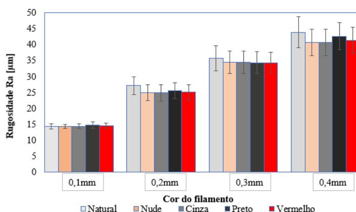
GRÁFICO 1. Resultados obtidos na rugosidade Ra para as diferentes alturas de camada.
