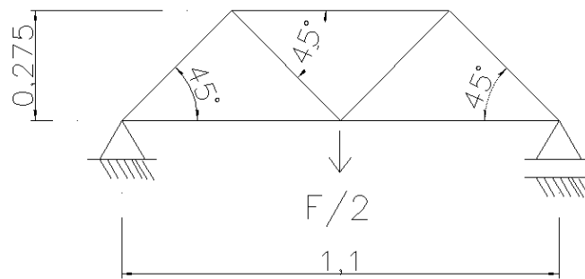
Figura 06- Modelo da treliça
