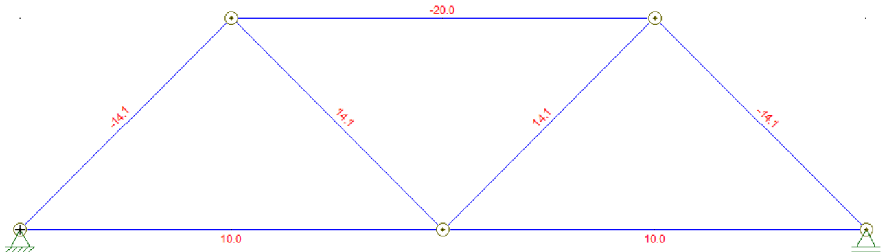
Figura 17- Esforços nas barras da treliça
