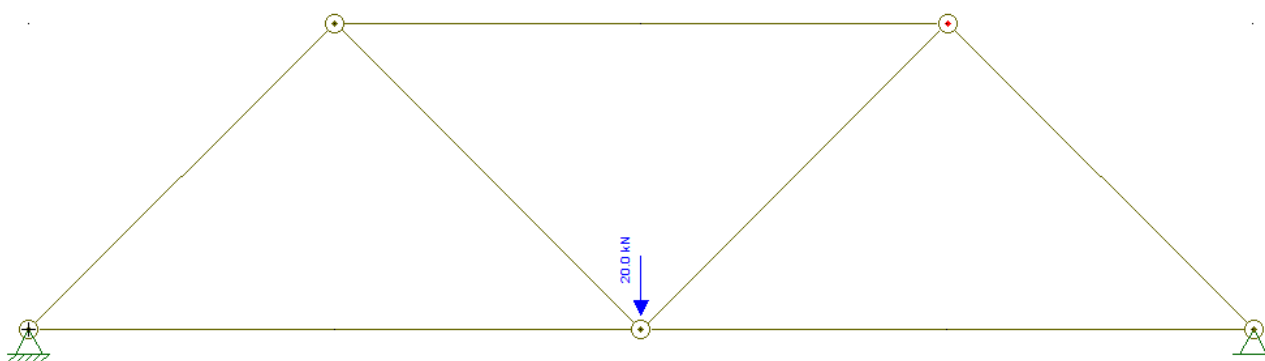
Figura 16- Treliça pronta para cálculo dos esforços
