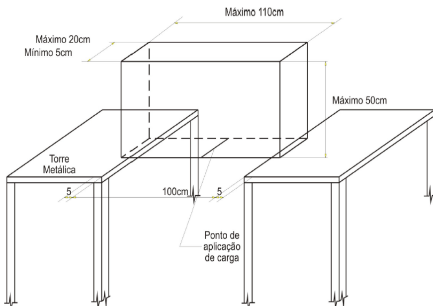
Figura 1- Esquema da ponte
