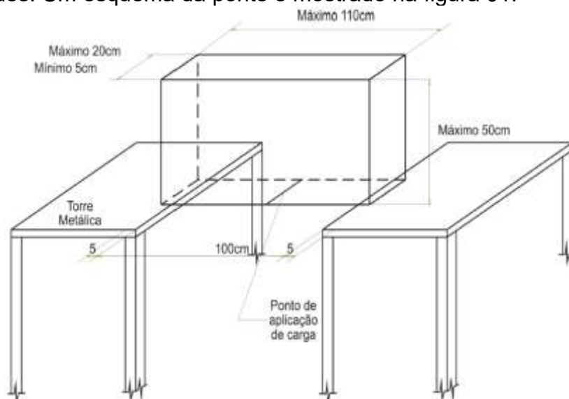
Figura 1- Esquema da ponte
